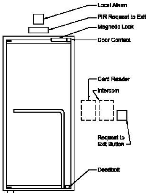
Door Type B - Frameless Single Door
