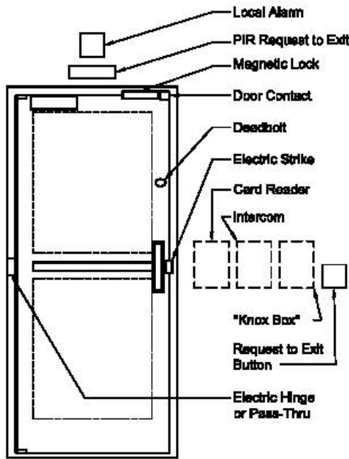
Door Type A - Single Opaque or Framed Glass Door
