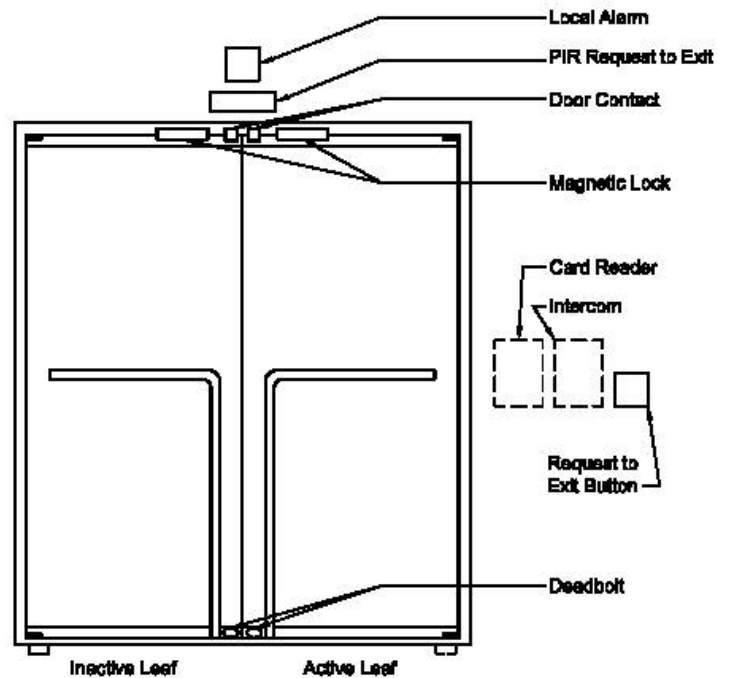
Door Type D - Frameless Pair of Doors
