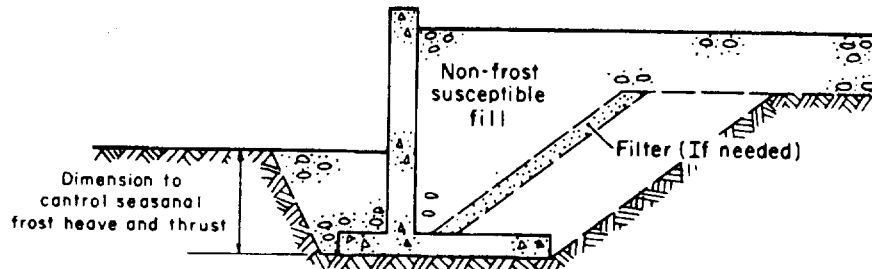
a. Counter fort wall
