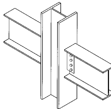
(d) Simple Shear Tab Connection
