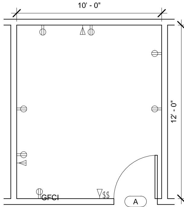
EYVF1 - FLOOR PLAN
